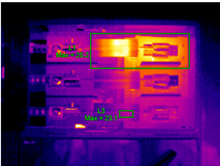
3-fázisú biztosíték túlmeledése
