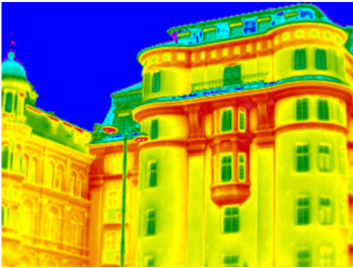
Épület hővesztés
