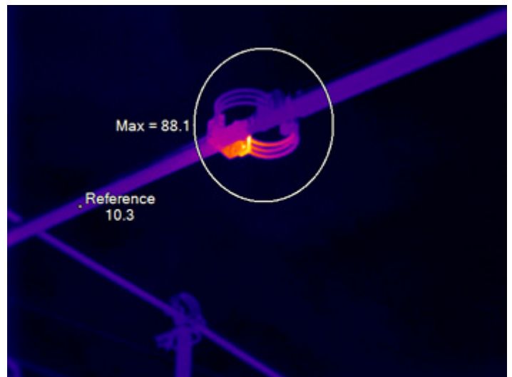
Villamosvezeték csatlakozási pontjának melegedése
